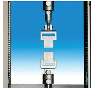
Morsetti H-test per prove di scollaggio.
