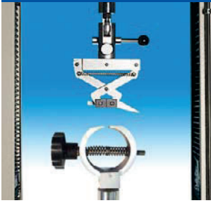
Coppia di morsetti per prove di stacco suola/tomaia.
