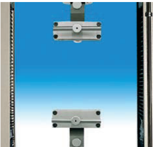
Morsetti con chiusura a vite per prove di trazione su: tessuti, finte pelli, pelli ecc.
