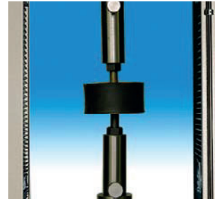
Dispositivo per prove di adesione compressione e su 4 quadranti, per antivibranti
