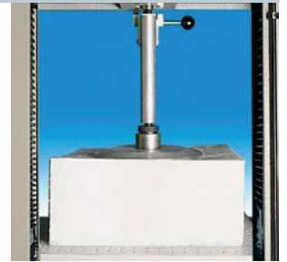
Dispositivo indentometro e per prove di portanza.
