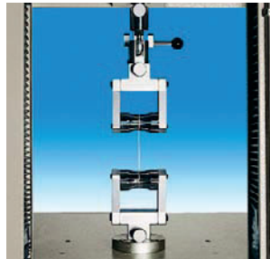
Morsetti autostringenti per prove di trazione su: cordonetti, corde, ecc.
