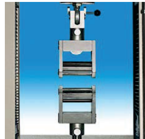
Morsetti autostringenti per prove di trazione su: nastri ecc.
