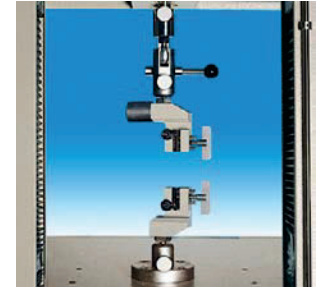
Morsetti per prove di trazione su: filati, cordonetti, ecc.
