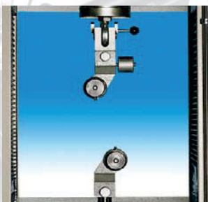
Morsetti per prove di trazione su: fili acciaio alta resistenza, ecc.
