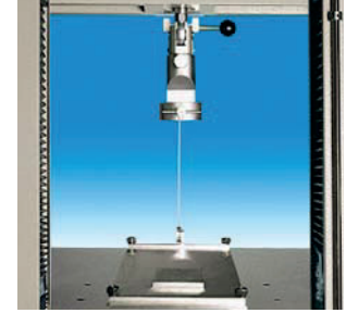
Dispositivo per prove di Friction Test: coefficiente di attrito statico e dinamico.
