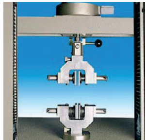
Morsetti con chiusura a vite per prove di trazione su: provini disassati ecc.
