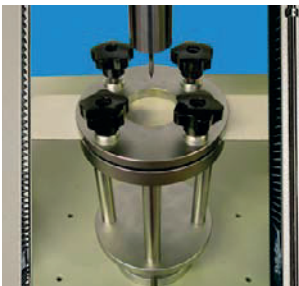
Dispositivo per prove di perforazione su: soles, solette, ecc.
