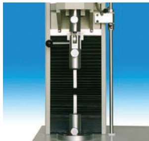
Dispositivo per prove di strappo su: pelli J.U.P.8.
