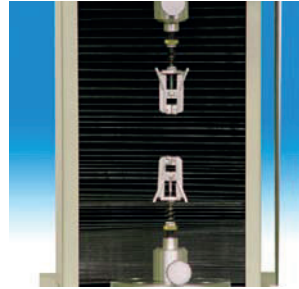
Morsetti per prove di trazione su: fibre e similari.
