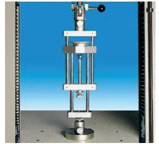
Dispositivo Persoz per prove: J.U.P. 9 su: pelli, tessuti, ecc.
