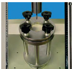
Dispositivo per prove di perforazione su: suole, solette, ecc.
