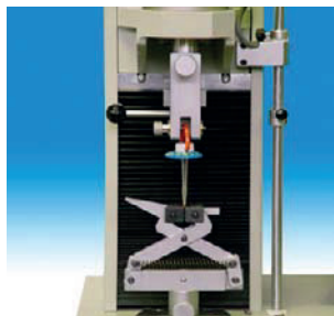
Dispositivo per prova tettarelle e succhiotti.
