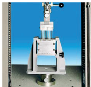
Dispositivo per prove di Kramer Shear.
