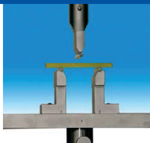
Dispositivo per prove di flessione a tre punti o a quattro punti.
