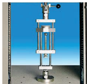
Dispositivo Persoz per prove: J.U.P. 9 su: pelli, tessuti, ecc.
